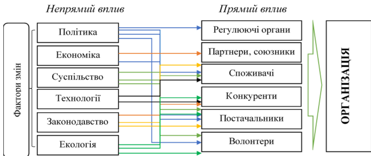
Рисунок 1.2 – Вплив середовища на організацію
